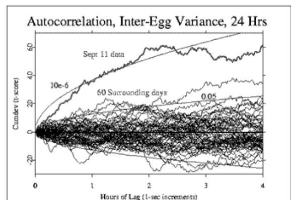
Рис. 1. Поведінка кумулятивних кривих у день теракту та в найближчі 60 днів
